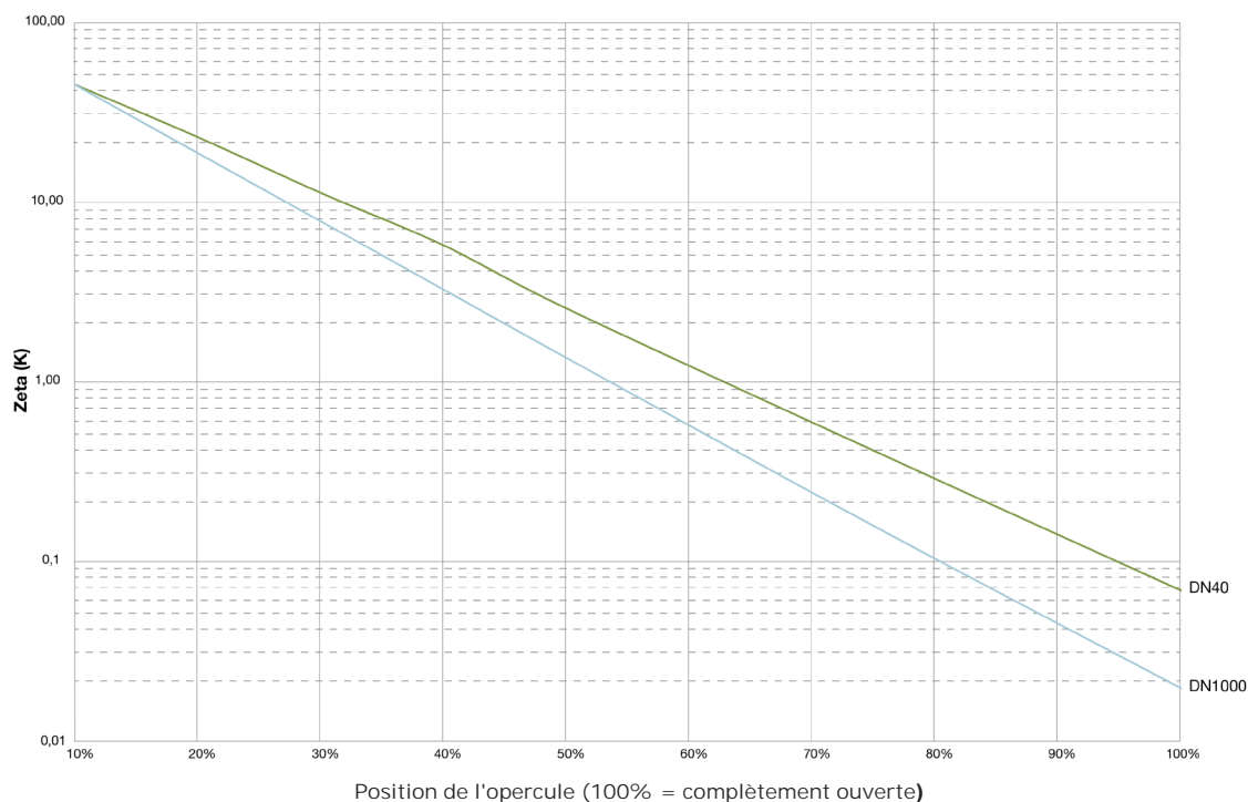
Valeurs Zeta (K) pour vanne opercule DN 40 - 1000
